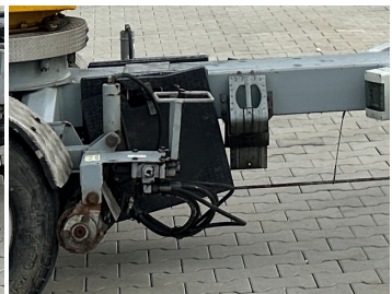
1550 EXB, 5373 CM-Unterlegplatten
