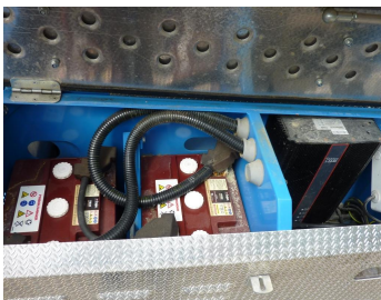
Gebr. Omme 2200 RBD - 8562 SLL - Batterieantrieb
